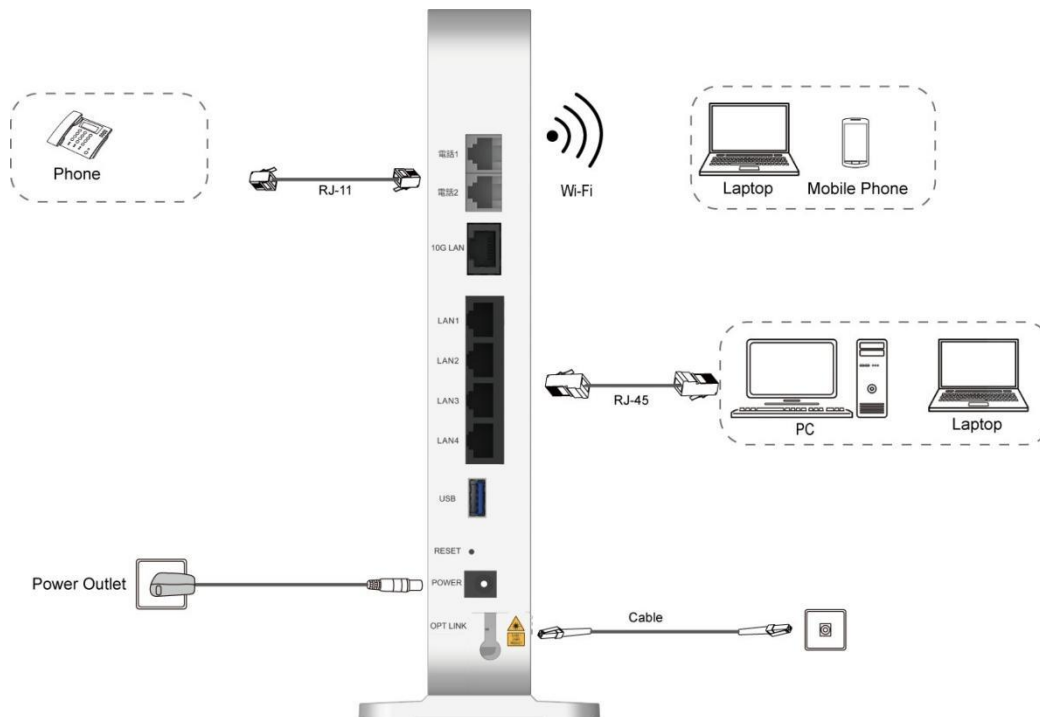
図 1-3 ケーブル・Wi-Fi 接続
