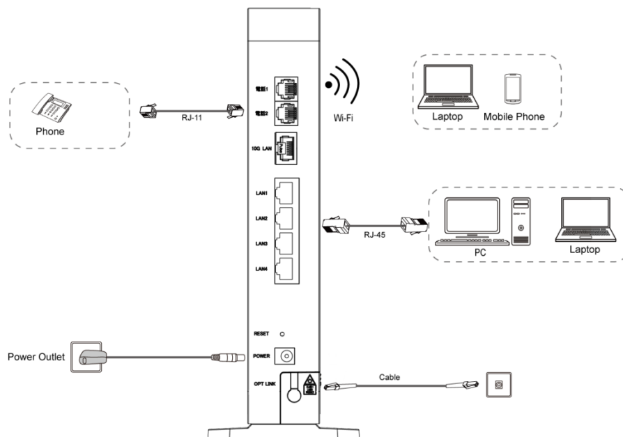
図 1-3 ケーブル・Wi-Fi 接続
